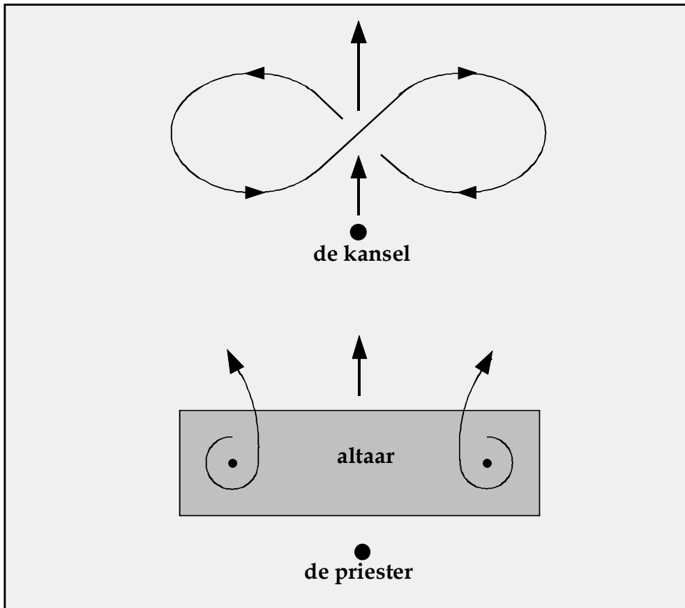
Vergelijking energieën bij lemniscaat en altaar.
